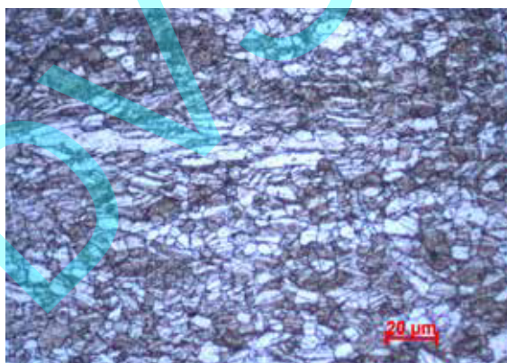
Bild 1 • Metallografischer Schliiff des Grundwerkstoffs AZ31 (geätzt in Pikrinsäure): \alpha -Mischkristalle mit vereinzelten mangan- und aluminiumreichen Ausscheidungen.
