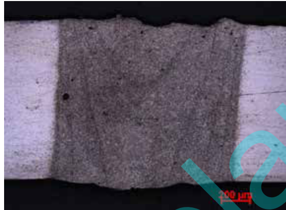
Bild 3 • Metallografischer Querschliff einer laserstrahlgeschweißten I-Naht am Stumpfstoß (Blechdicke 1 \text{ mm} ).
