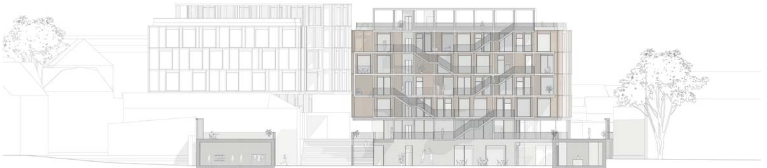
Westansicht Haus 2 M 1_200
